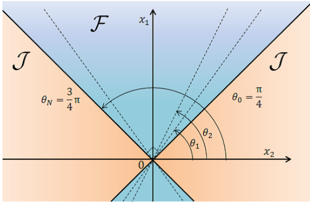
Fig. 2 フローセット \mathcal{F} の x_1 - x_2 平面における断面
